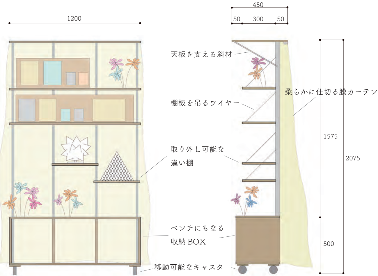
立面図 S1：20
